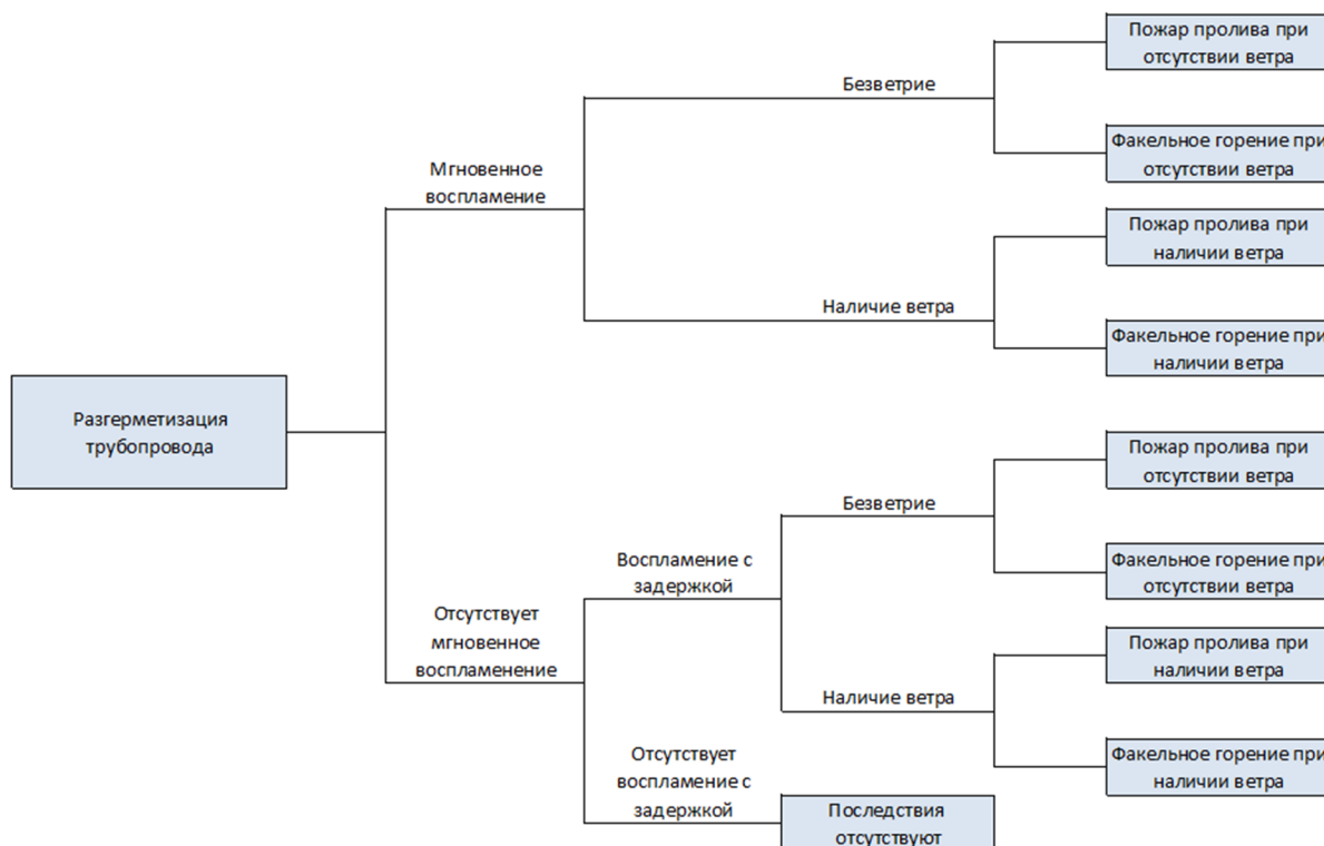
Рис. 3.5.1. Дерево событий развития пожароопасных ситуаций на продуктопроводе
