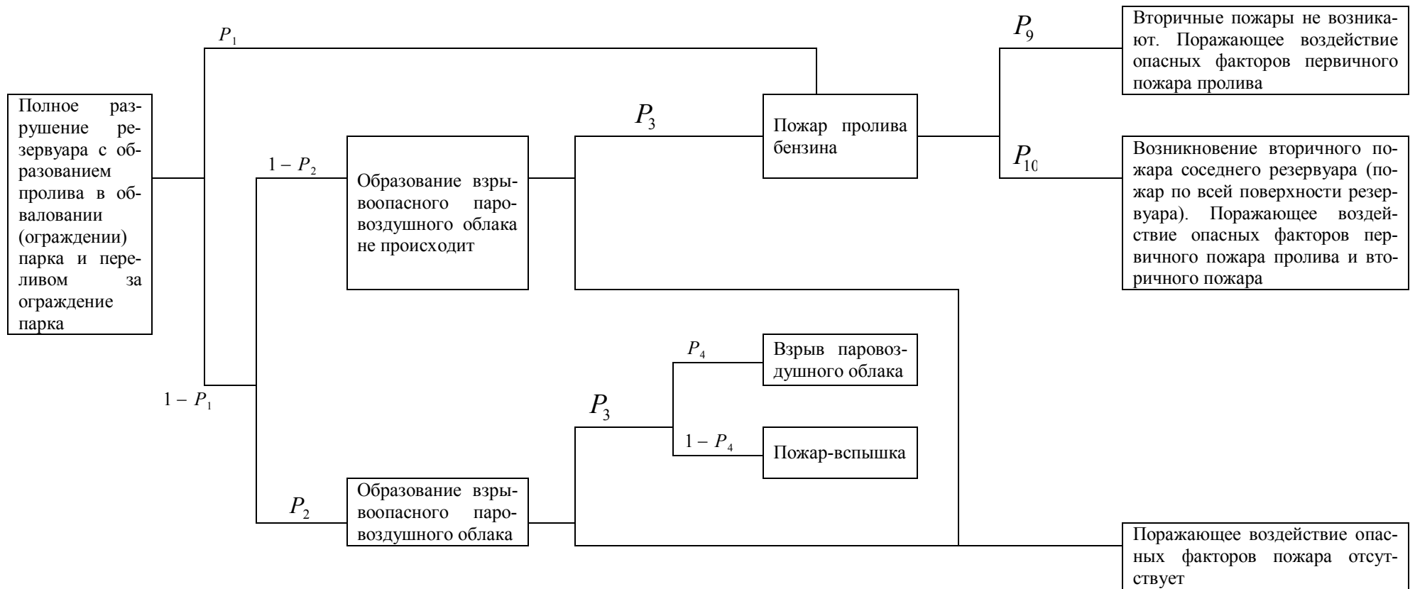
Рис. 3.2.2. Дерево событий при возникновении и развитии пожароопасной ситуации, связанной с полным разрушением одного из резервуаров рассматриваемого резервуарного парка
