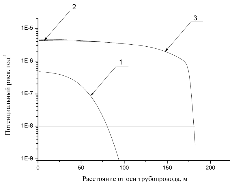
Рис. 3.5.6. Зависимость потенциального пожарного риска от расстояния от оси трубопровода и вклад k -го сценария аварии в величину суммарного потенциального пожарного риска на участке перехода рассматриваемого продуктопровода через водную преграду. 1 – факельное горение; 2 – пожар пролива; 3 – суммарный потенциальный пожарный риск; 4 – предельное допустимое значение индивидуального пожарного риска для населения, регламентированное [3]
