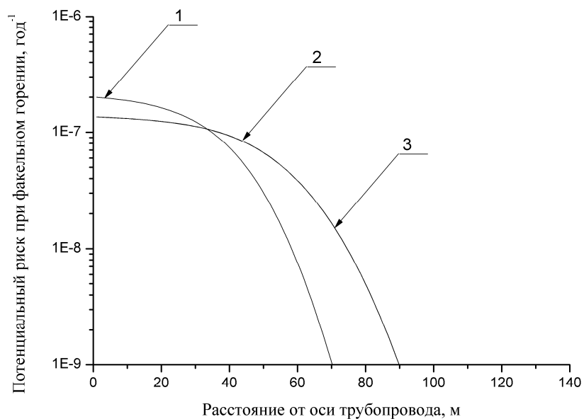
Рис. 3.5.5. Зависимость потенциального пожарного риска факельного горения от расстояния от оси трубопровода для различных типов повреждений рассматриваемого продуктопровода 1 – «свищ»; 2 – «трещина»; 3 – «гильотинный разрыв»
