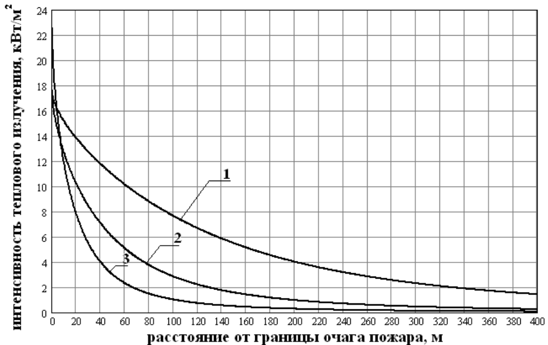
Рис. 3.2.5. Зависимости интенсивности теплового излучения пожара пролива бензина от расстояния до границы очага пожара, при площади очага:
